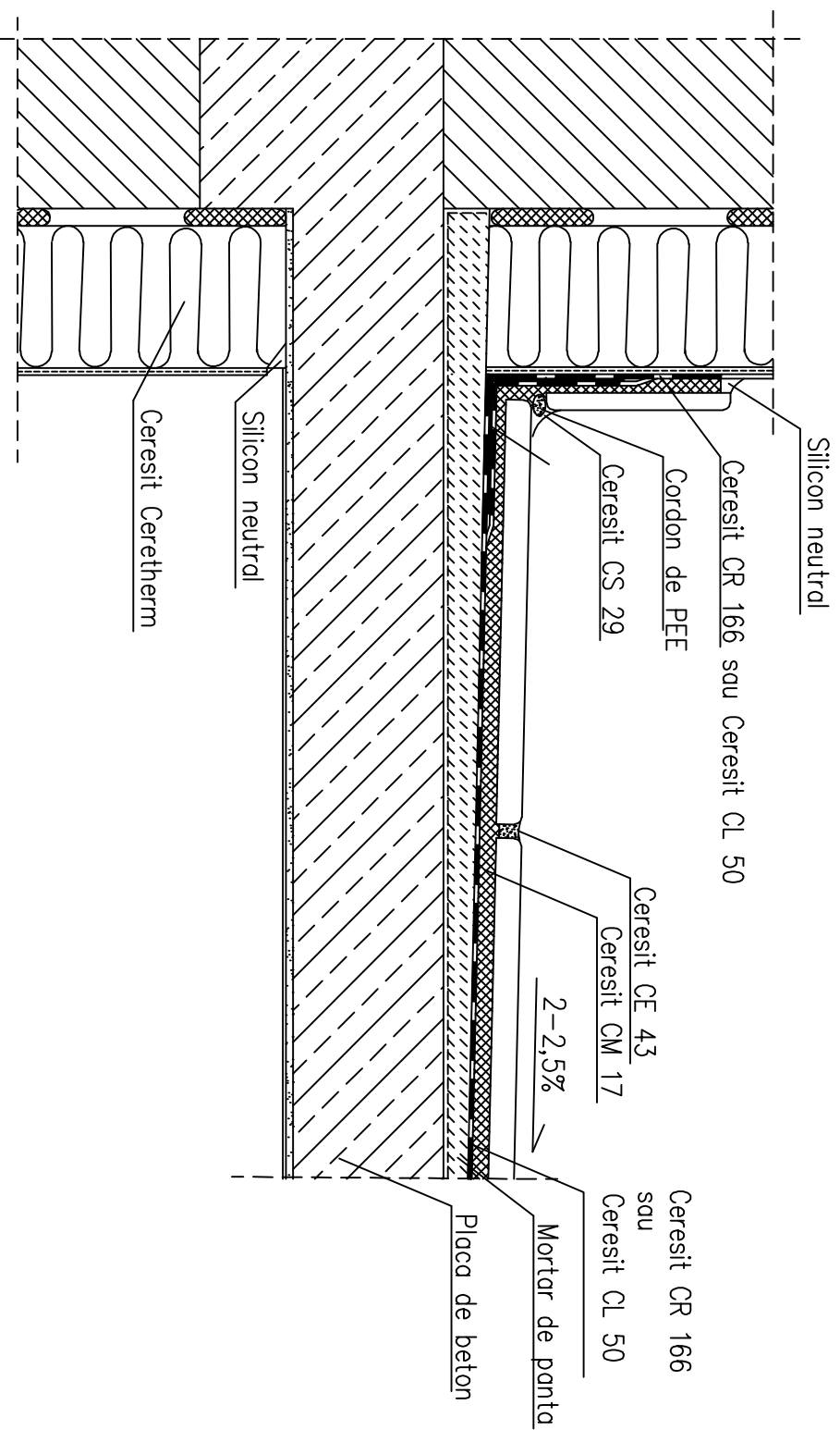
Fig. 1.2 Imbinarea dintre placa balconului si perete
